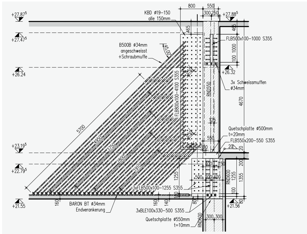
An den Vollstahlkern angeschweisst sind ein Stahlschwert und ein Bündel geneigter, hochduktiler Schraubarmierungseisen mit Kopfbolzendübeln, welche die ungeheuren Kräfte des hier lastenden Mitteltrakts in die Vertikale zwingen.
